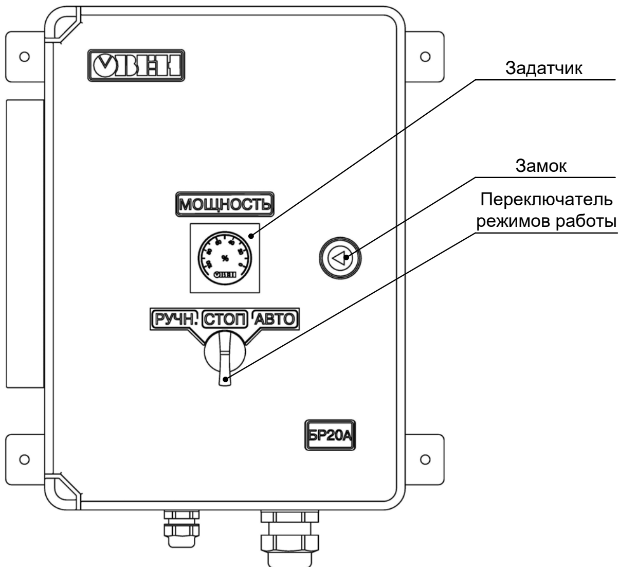
Рисунок 4.2 – Внешний вид дверцы
