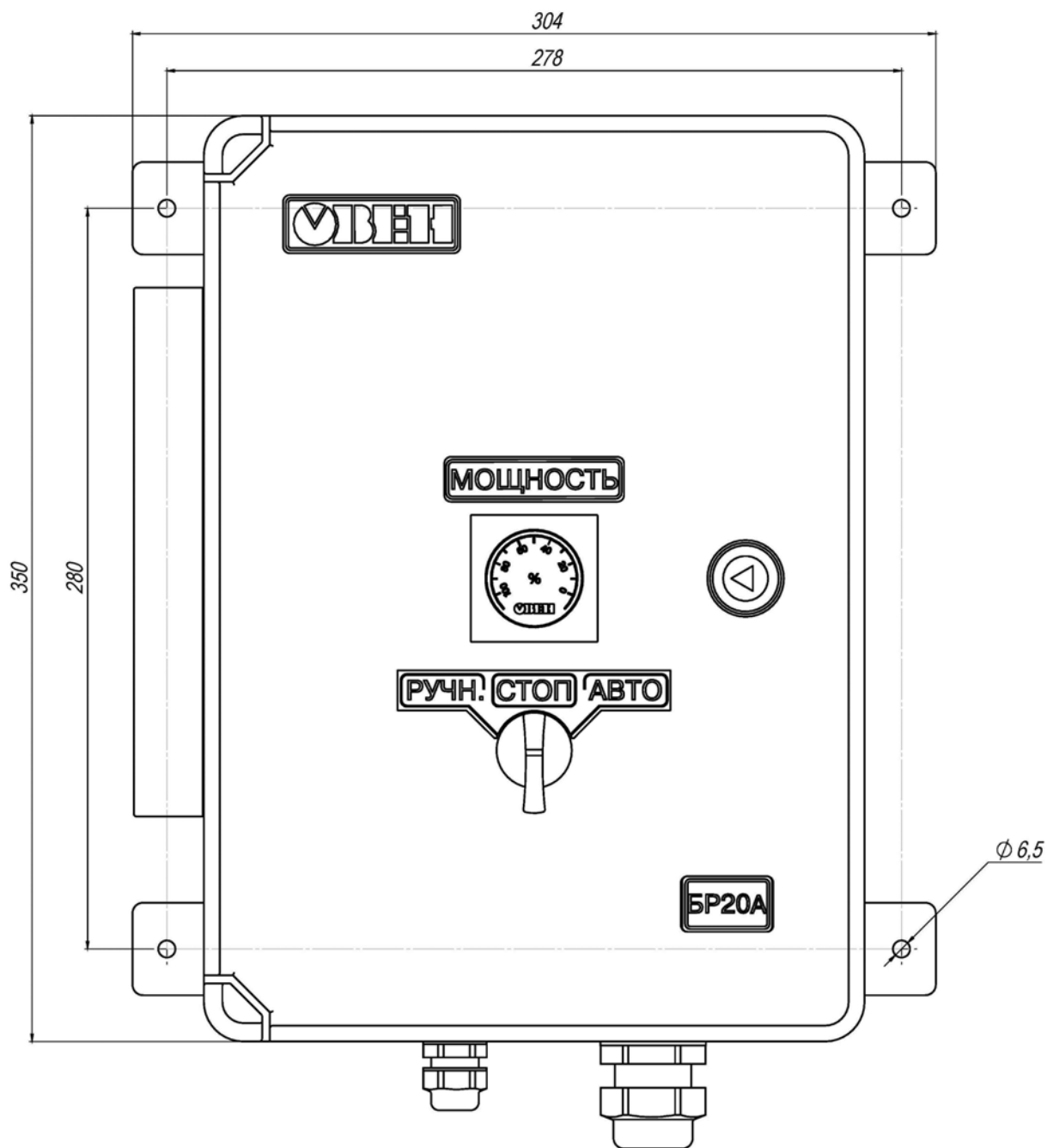
Рисунок В.1 – Габаритный чертеж вид спереди
