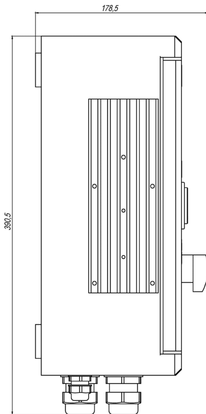
Рисунок В.2 – Габаритный чертеж вид сбоку
