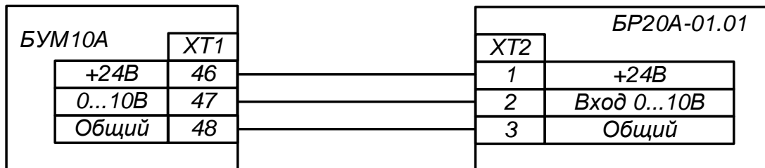
Рисунок А.3 – Подключение к БУМ10А для регулирования скорости вращения однофазных вентиляторов
