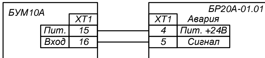
Рисунок А.4 – Подключение к БУМ10А для идентификации перехода блока BR20A-01.01 в режим РУЧНОЙ или СТОП
