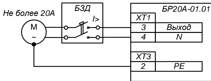
Рисунок А.2 – Подключение нагрузки
