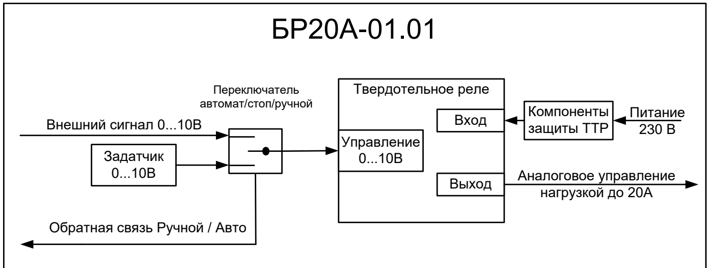
Рисунок 4.1 – Функциональная схема блока
